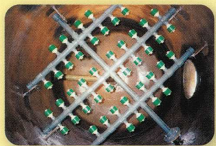
KSH Distribuidor con toberas
